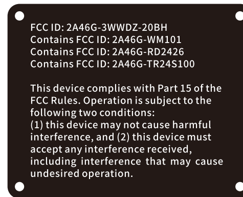
轮廓图 (白色图案与文字是需要镭雕的内容)
