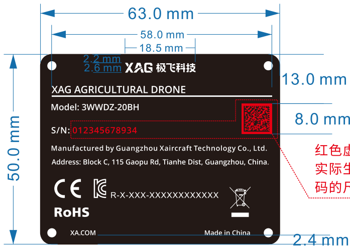
尺寸图
