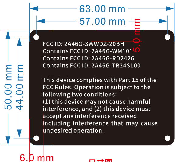
尺寸图
