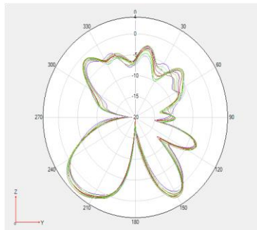
Phi 90 2D图
