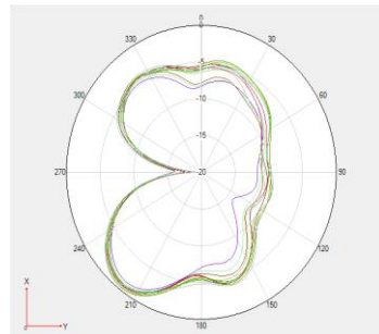
Theta 90 2D图
