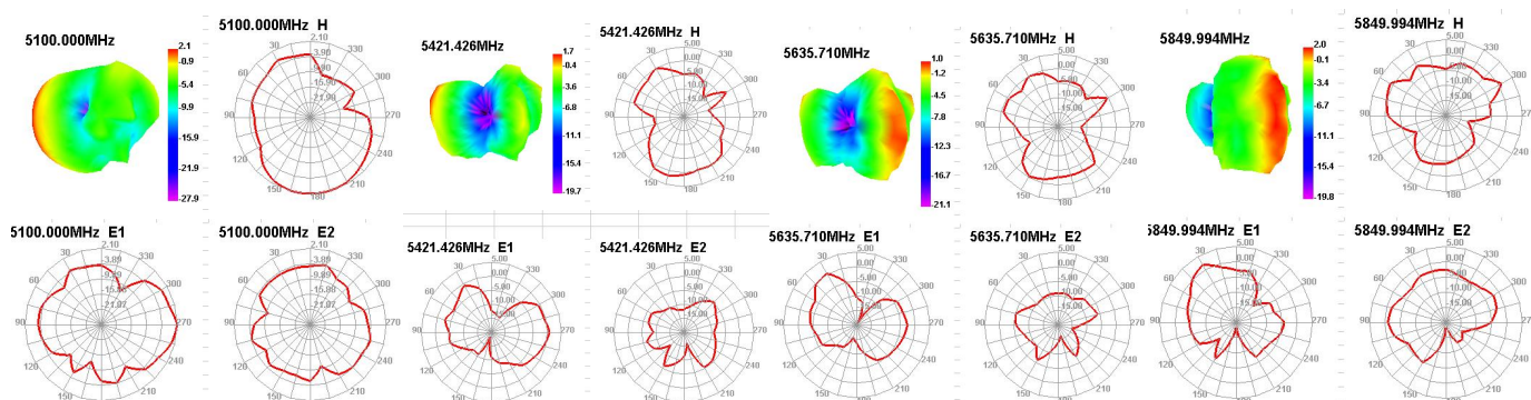
5100.00MHz - 5850.00MHz Gain
