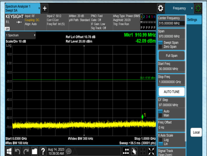
11B-Ant1-2412-30~1000
