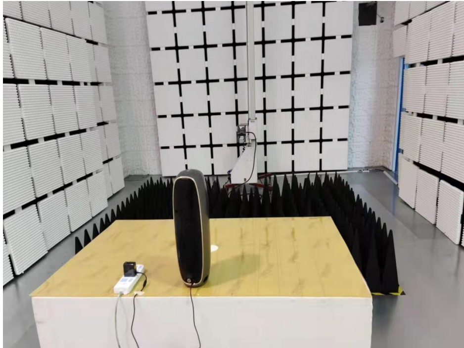
RSE 1GHz-18GHz
