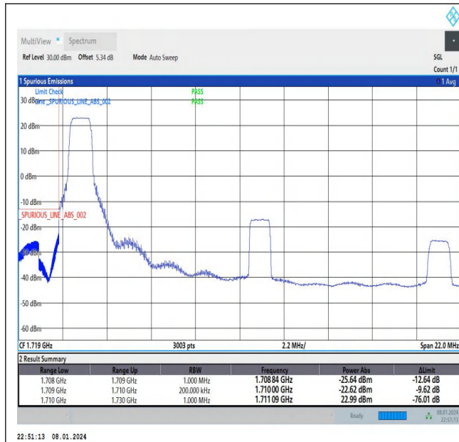
Band66_20MHz_QPSK_132072_1RB#0
