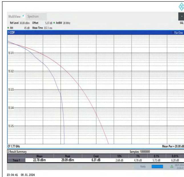
Band66-20MHz-QPSK-132572-1RB#0-PASS
