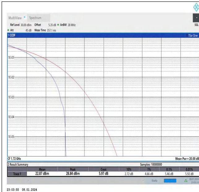
Band66-20MHz-QPSK-132072-1RB#0-PASS
