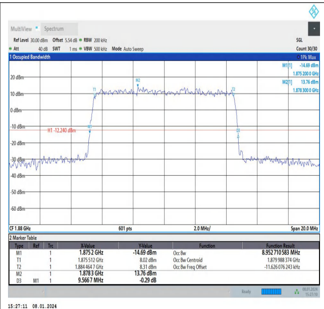
Band2-10MHz-16QAM-18900-50RB#0-PASS
