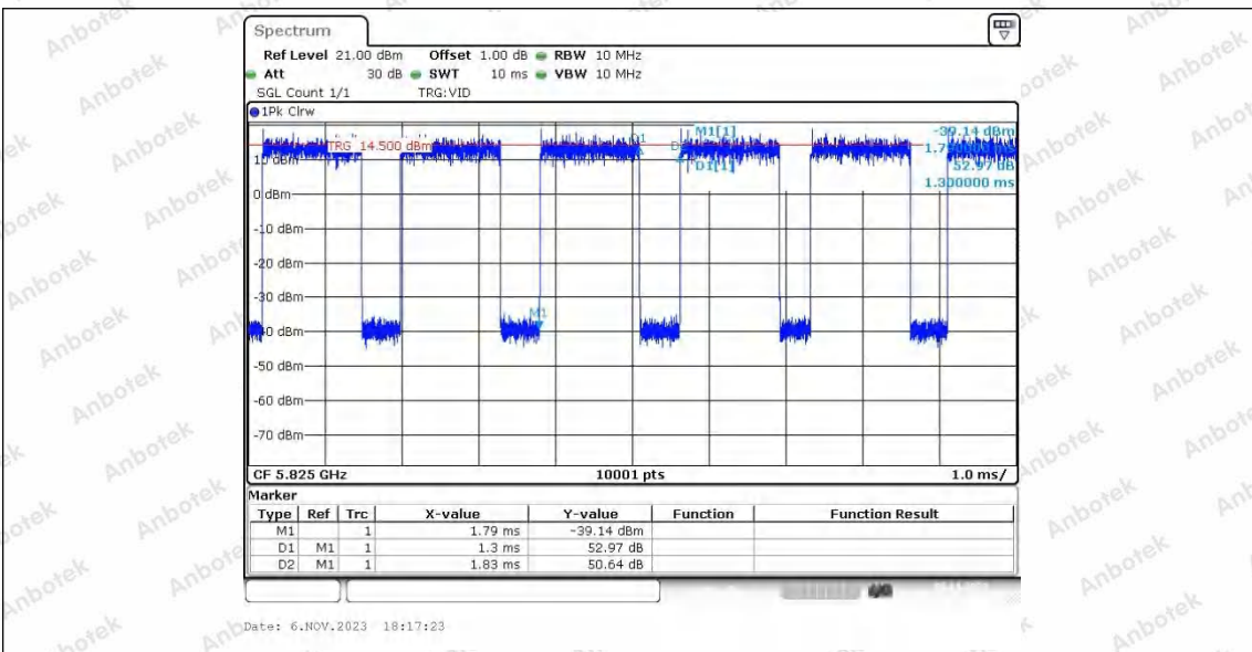
11N20SISO_Ant2_5825
