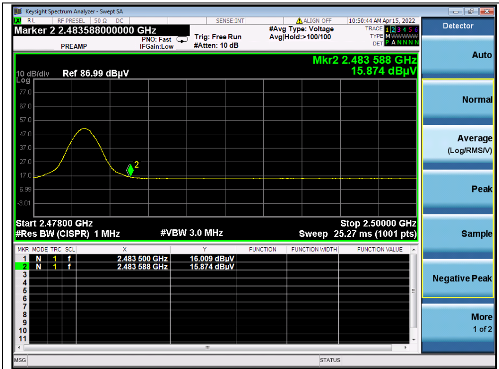
(AVERAGE, Channel 81)
