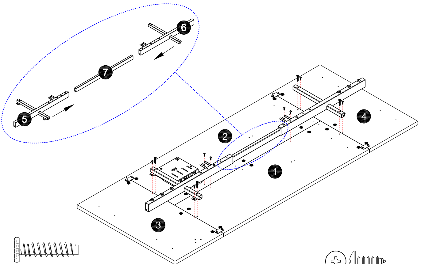
F. 6x28mm Screw - 4
