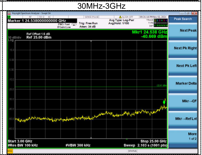
3G-25G
