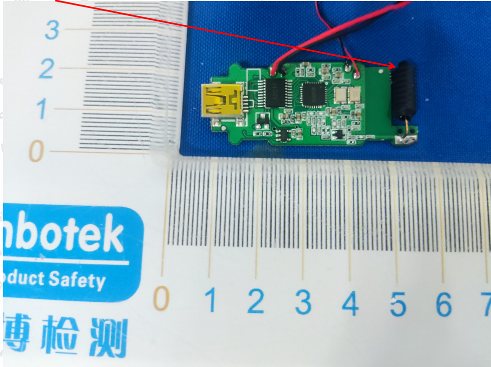
RX ANT
