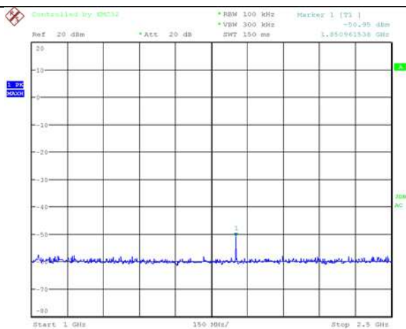
1-2.5GHz
