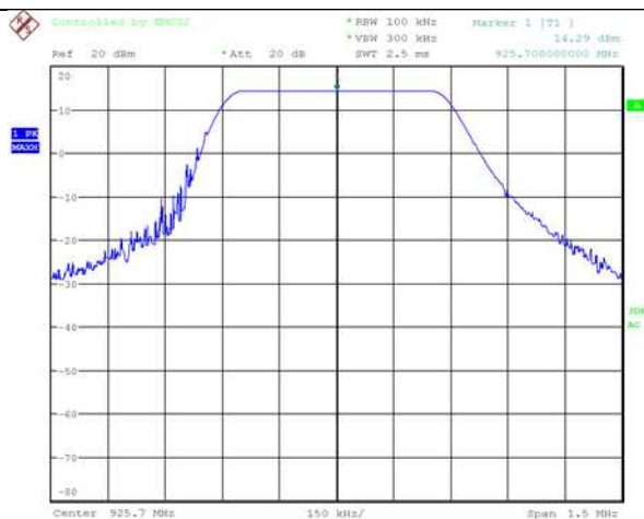
Fundamental
