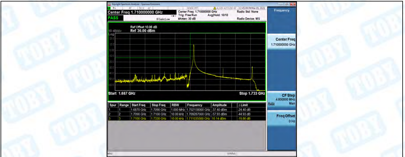
Band66-20MHz-QPSK-132072-1RB#99
