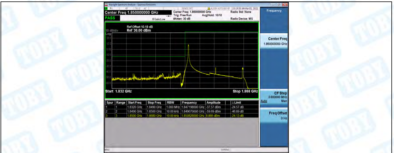
Band2-15MHz-16QAM-18675-1RB#74
