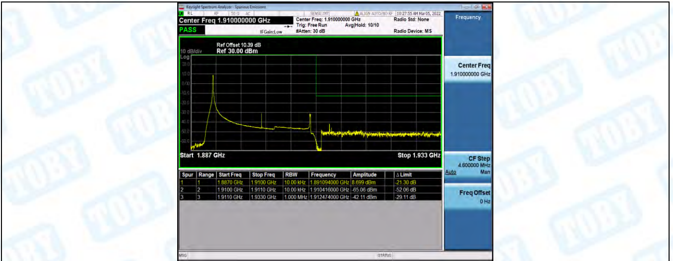
Band2-20MHz-16QAM-19100-1RB#99
