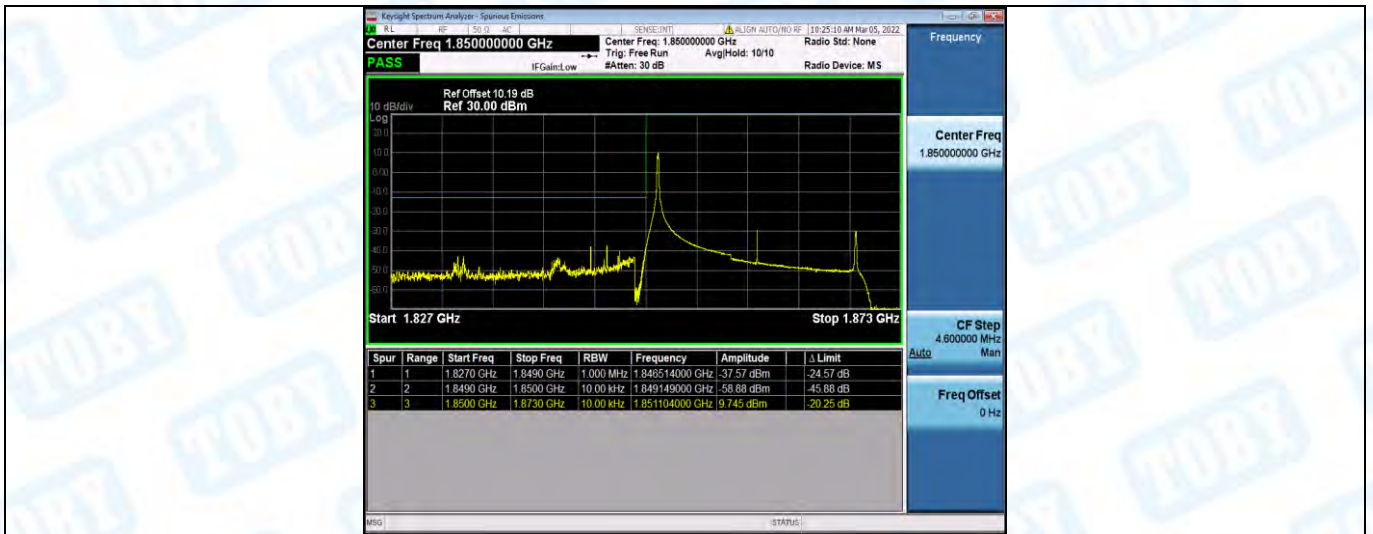
Band2-20MHz-QPSK-18700-1RB#99
