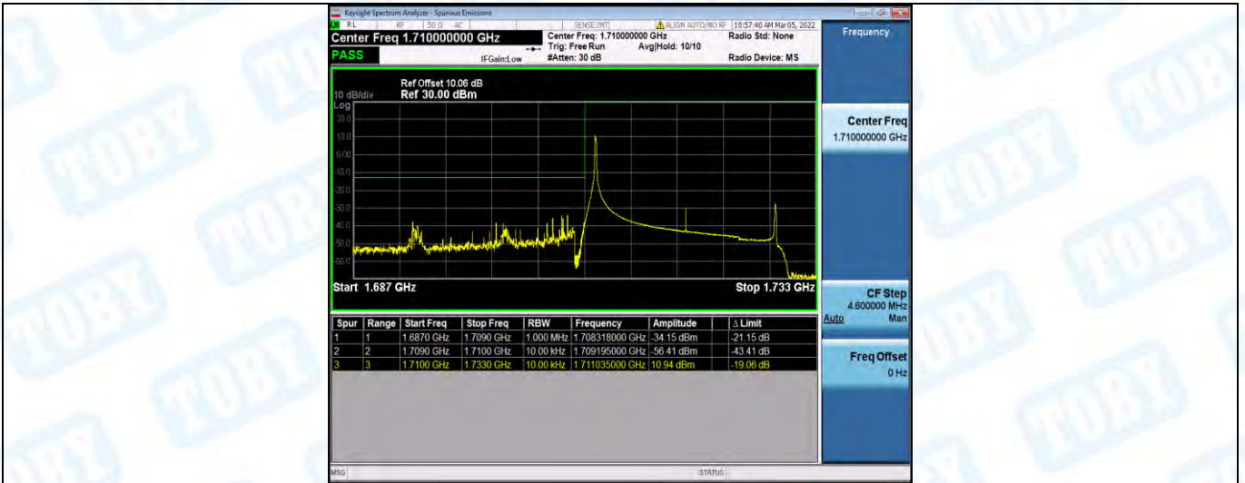
Band4-20MHz-QPSK-20050-1RB#99
