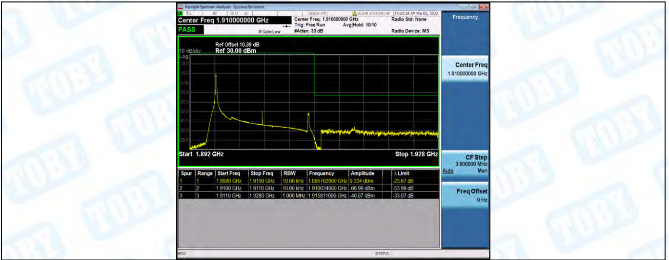
Band2-15MHz-16QAM-19125-1RB#74
