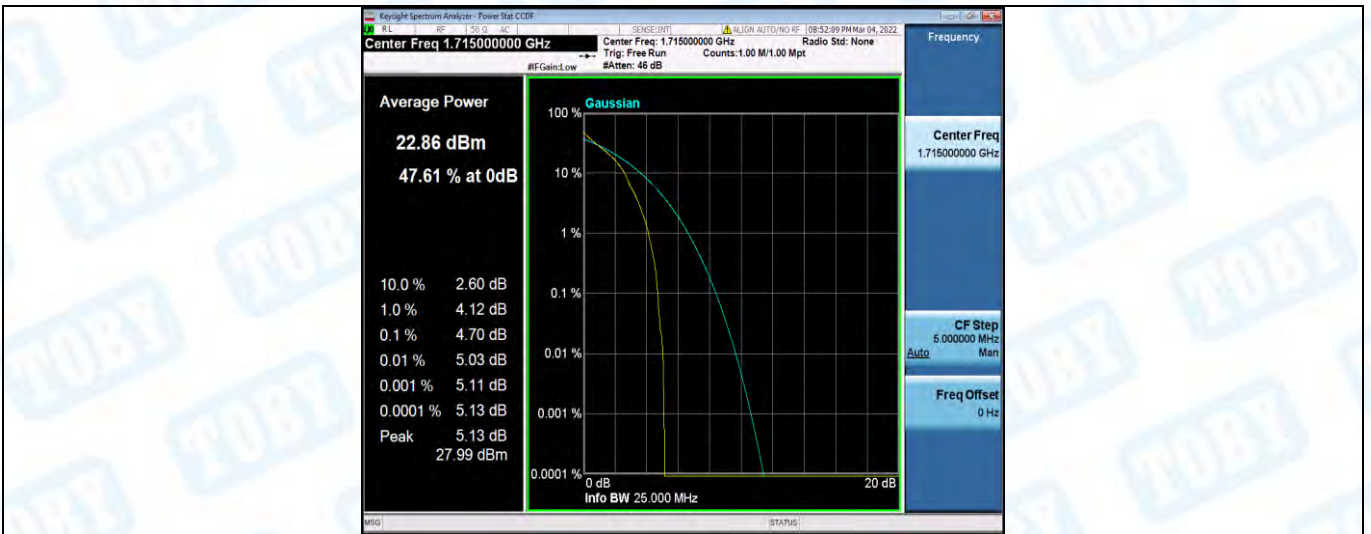
Band4-10MHz-QPSK-20000-50RB#0
