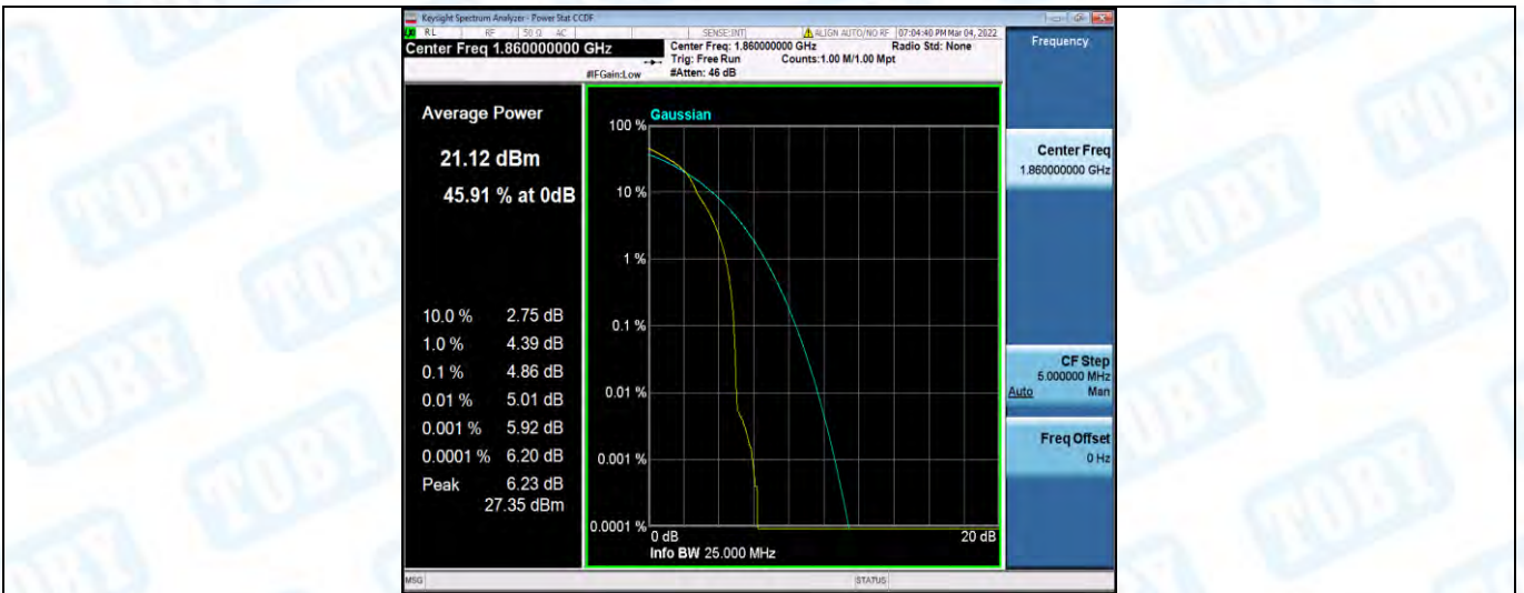
Band2-20MHz-16QAM-18700-100RB#0
