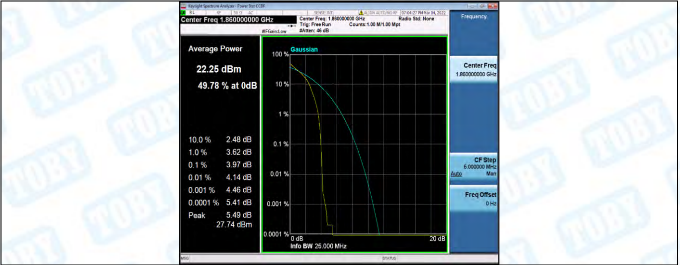
Band2-20MHz-QPSK-18700-100RB#0
