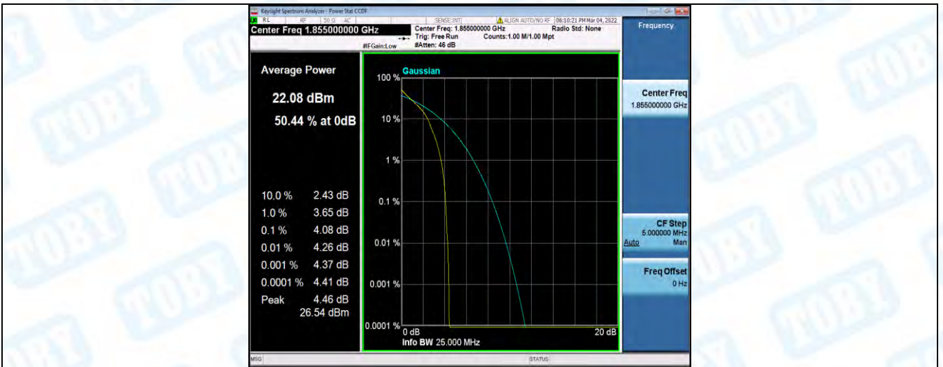
Band2-10MHz-QPSK-18650-50RB#0
