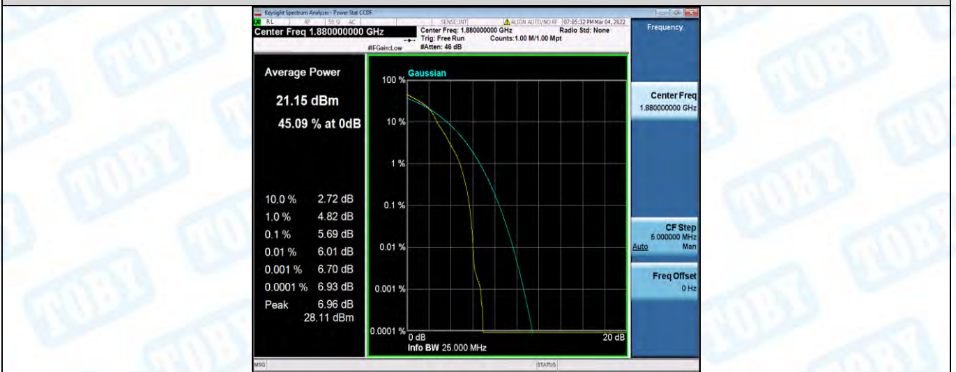
Band2-20MHz-16QAM-18900-100RB#0
