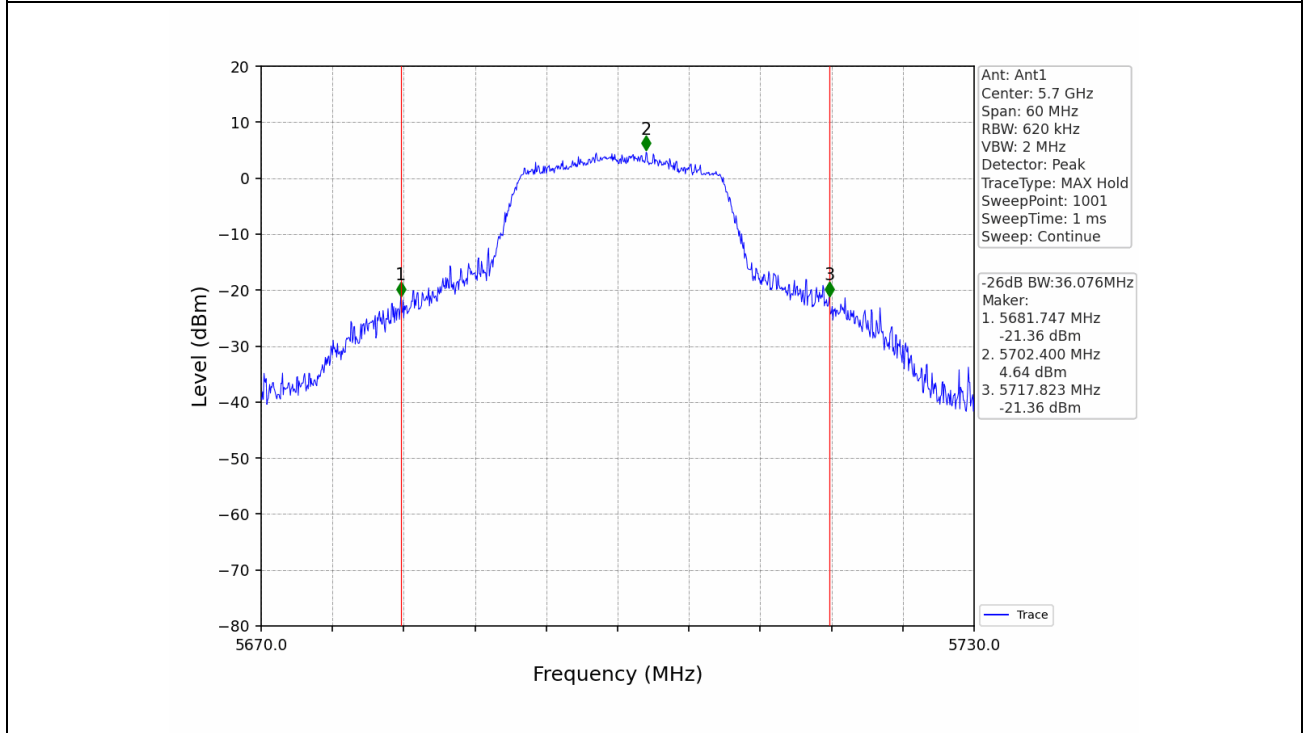
802.11ac(VHT20)_HCH_5700MHz_Ant1_NTNV
