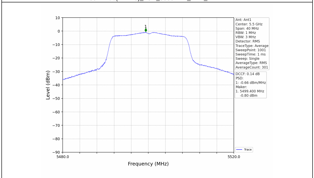
802.11ac(VHT20)_LCH_5500MHz_Ant1_NTNV
