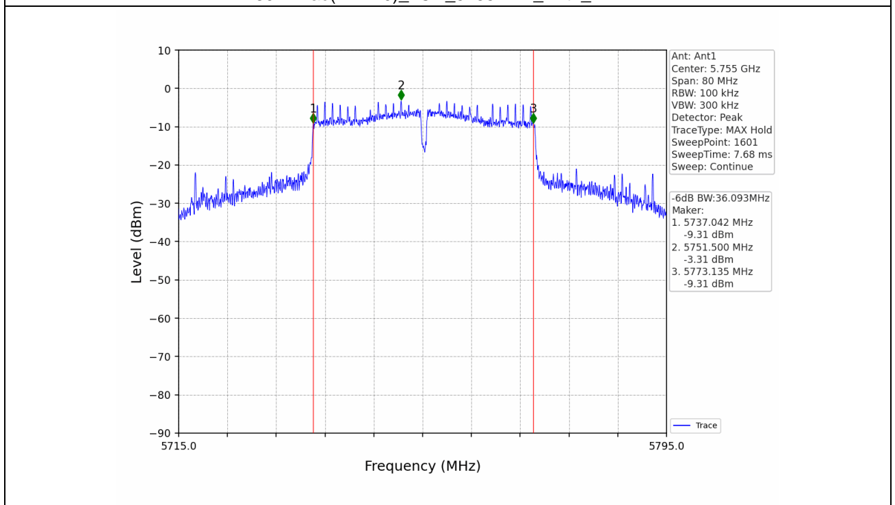
802.11ac(VHT40)_LCH_5755MHz_Ant1_NTNV
