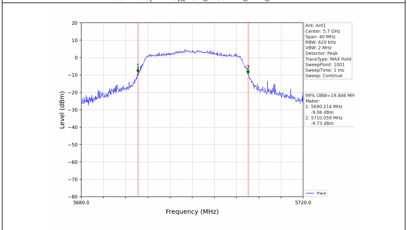
802.11ac(VHT20)_HCH_5700MHz_Ant1_NTNV
