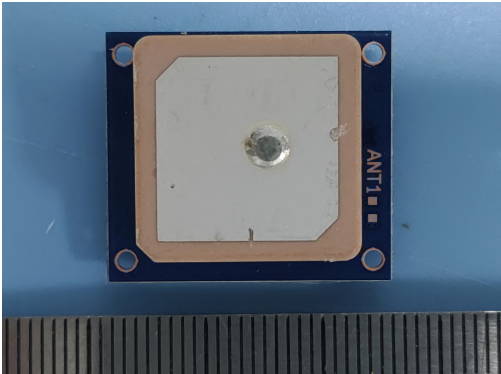
GPS Antenna
