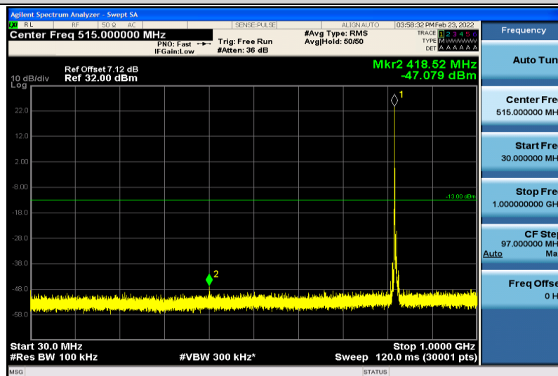
Band18-5MHz-QPSK-23895-1RB#0-30~1000MHz
