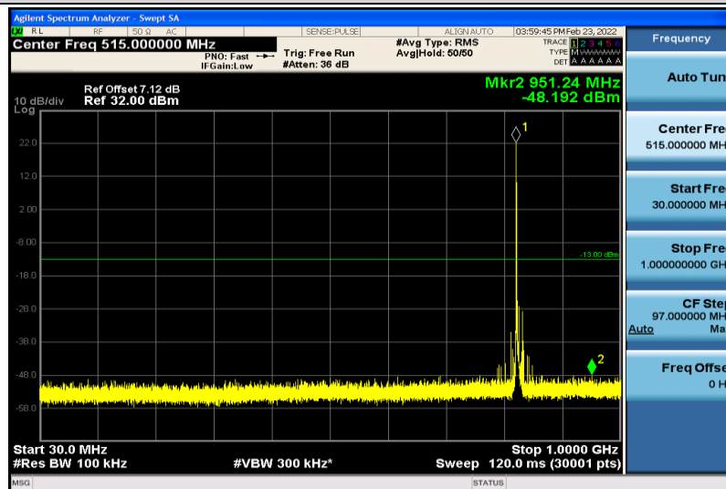
Band18-5MHz-QPSK-23915-1RB#0-30~1000MHz
