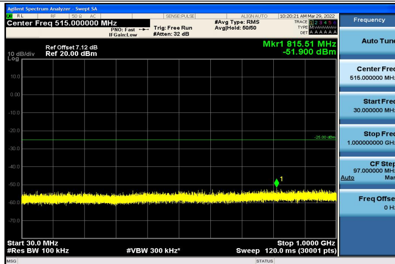
Band41-5MHz-QPSK-41215-1RB#0-30~1000MHz
