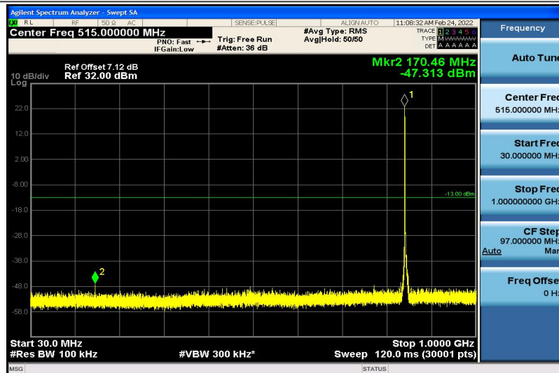
Band26-5MHz-QPSK-27015-1RB#0-30~1000MHz
