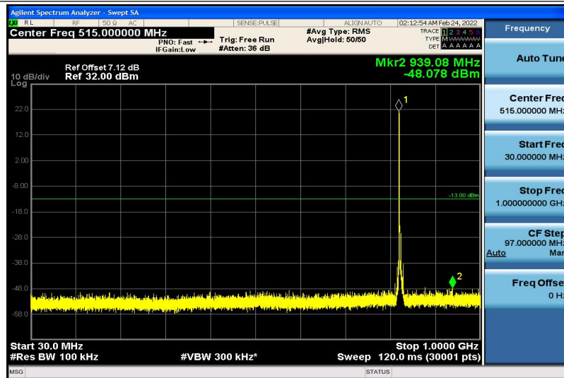
Band18-5MHz-QPSK-23965-1RB#0-30~1000MHz
