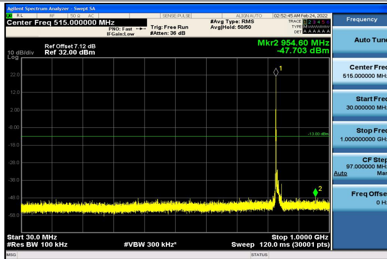
Band19-10MHz-QPSK-24050-1RB#0-30~1000MHz
