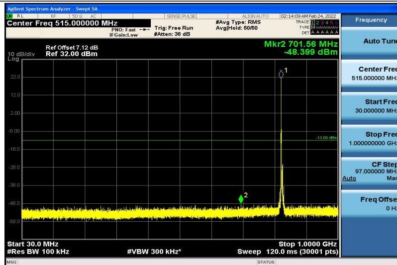
Band18-5MHz-QPSK-23970-1RB#0-30~1000MHz
