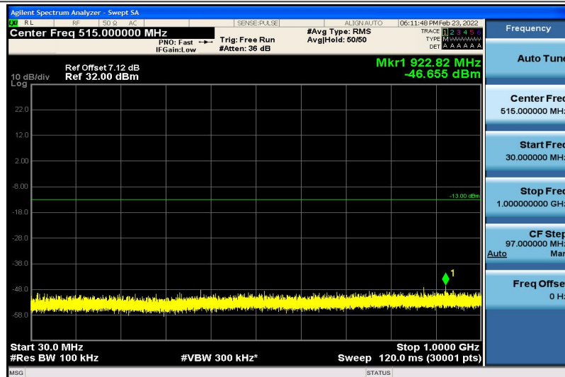
Band2-20MHz-QPSK-18900-1RB#0-30~1000MHz
