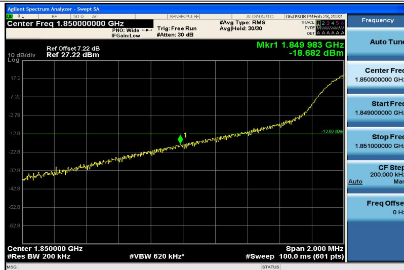
Band2-20MHz-16QAM-18700-1RB#0
