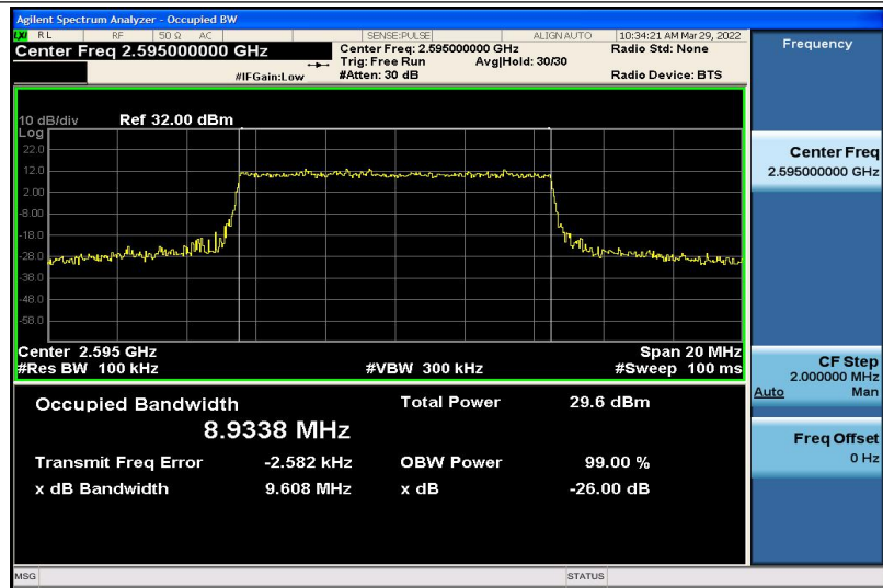
Band41-10MHz-QPSK-40640-50RB#0-8.9338
