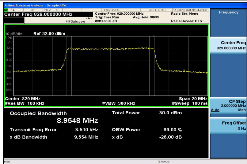
Band26-10MHz-QPSK-26840-50RB#0-8.9548
