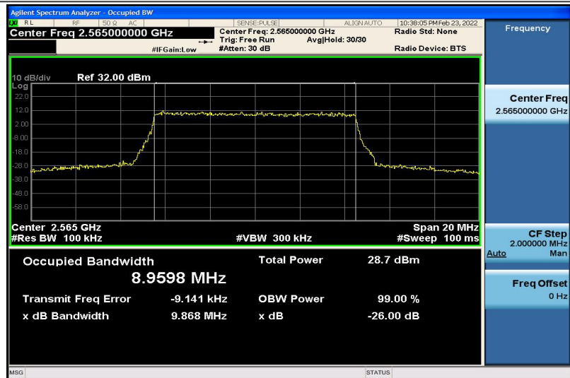
Band7-10MHz-QPSK-21400-50RB#0-8.9598
