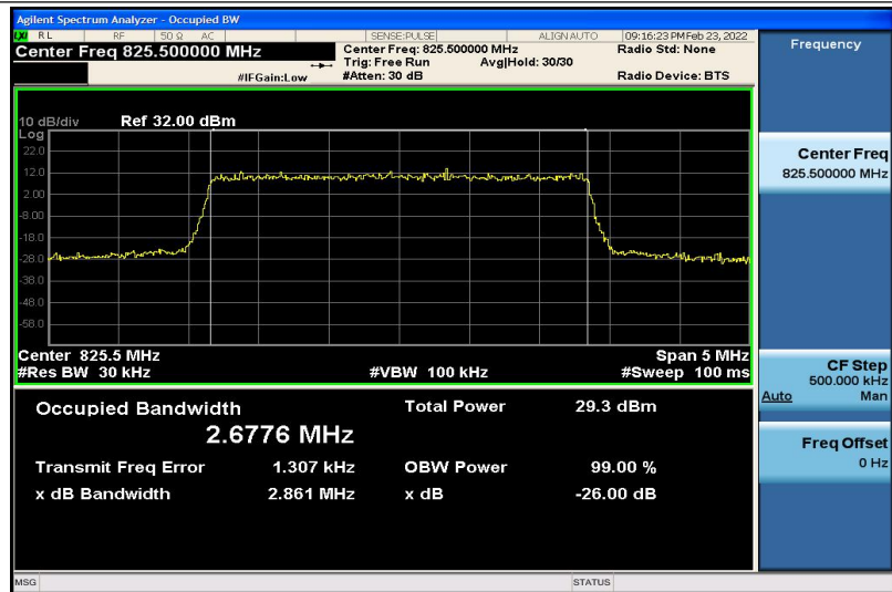
Band5-3MHz-QPSK-20415-15RB#0-2.6776
