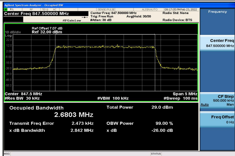
Band5-3MHz-QPSK-20635-15RB#0-2.6803
