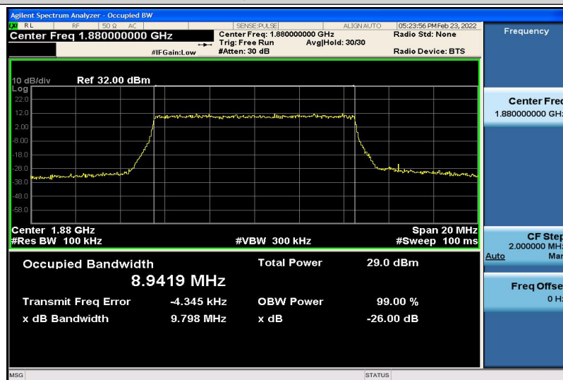
Band2-10MHz-QPSK-18900-50RB#0-8.9419
