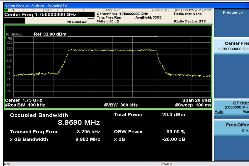
Band4-10MHz-QPSK-20350-50RB#0-8.9590
