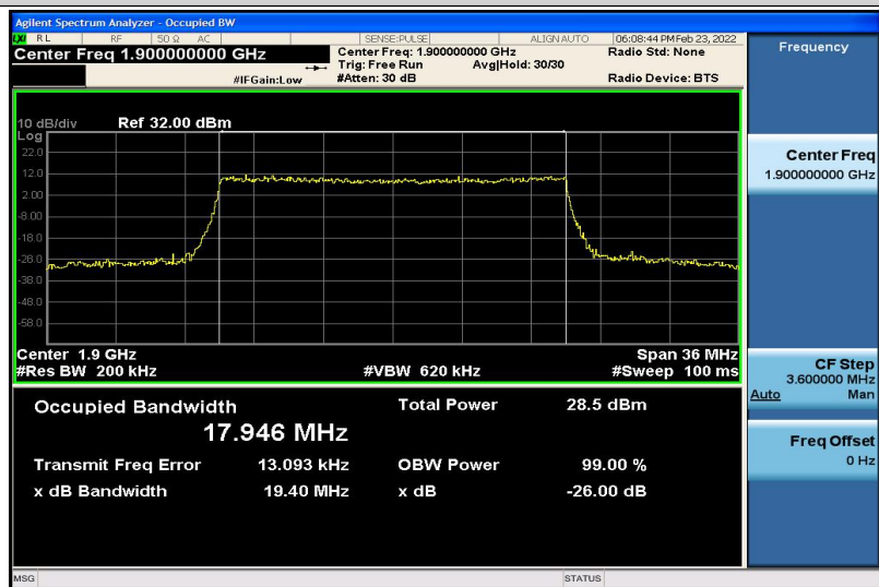
Band2-20MHz-16QAM-19100-100RB#0-17.946
