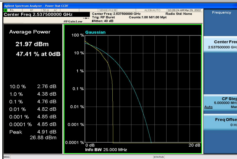
Band41-5MHz-QPSK-40065-1RB#0
