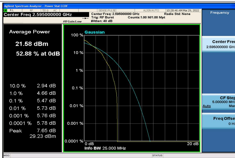
Band41-5MHz-QPSK-40640-1RB#0
