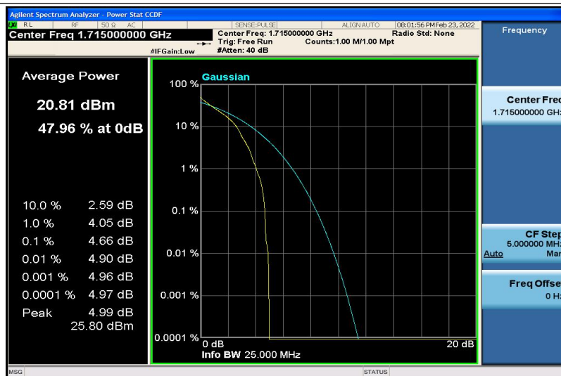
Band4-10MHz-QPSK-20000-1RB#0
