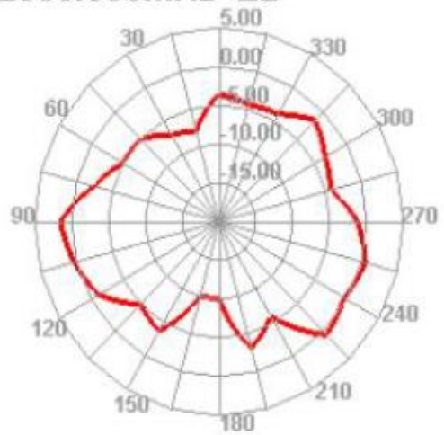
2500.000MHz E2
