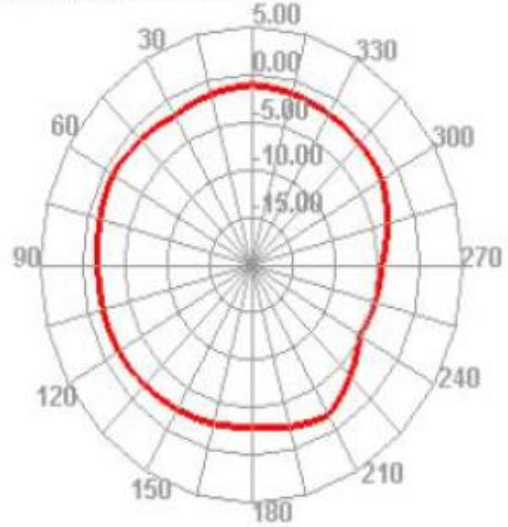
2450.000MHz H
