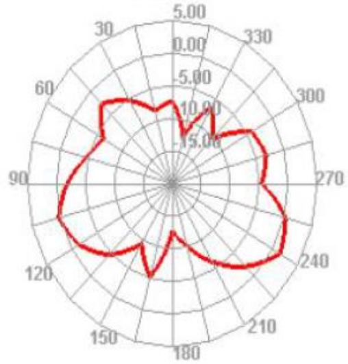
2450.000MHz E2
