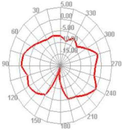
2450.000MHz E1
