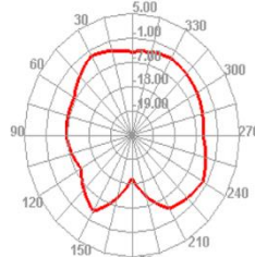
2500.000MHz E2
