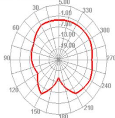
2450.000MHz E2
