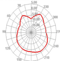
2500.000MHz E2
