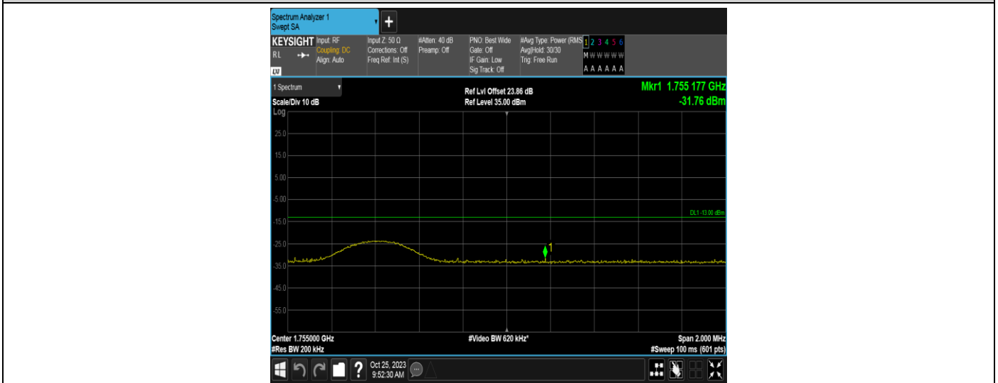
Band4-10MHz-QPSK-20350-1RB#0
