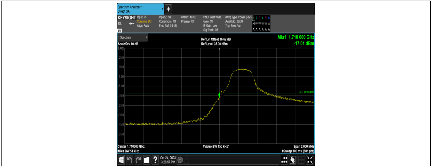
Band4-3MHz-QPSK-19965-1RB#14
