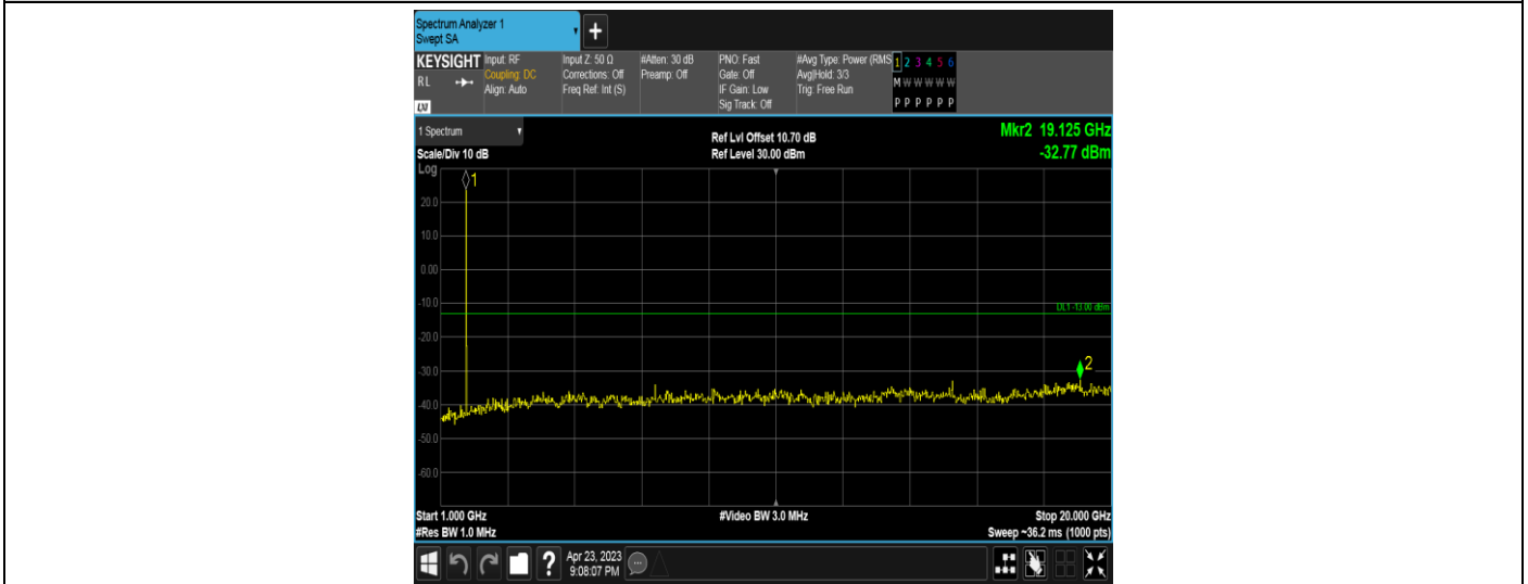
Band4-10MHz-QPSK-20175-1RB#0-Range2:1000~20000MHz
