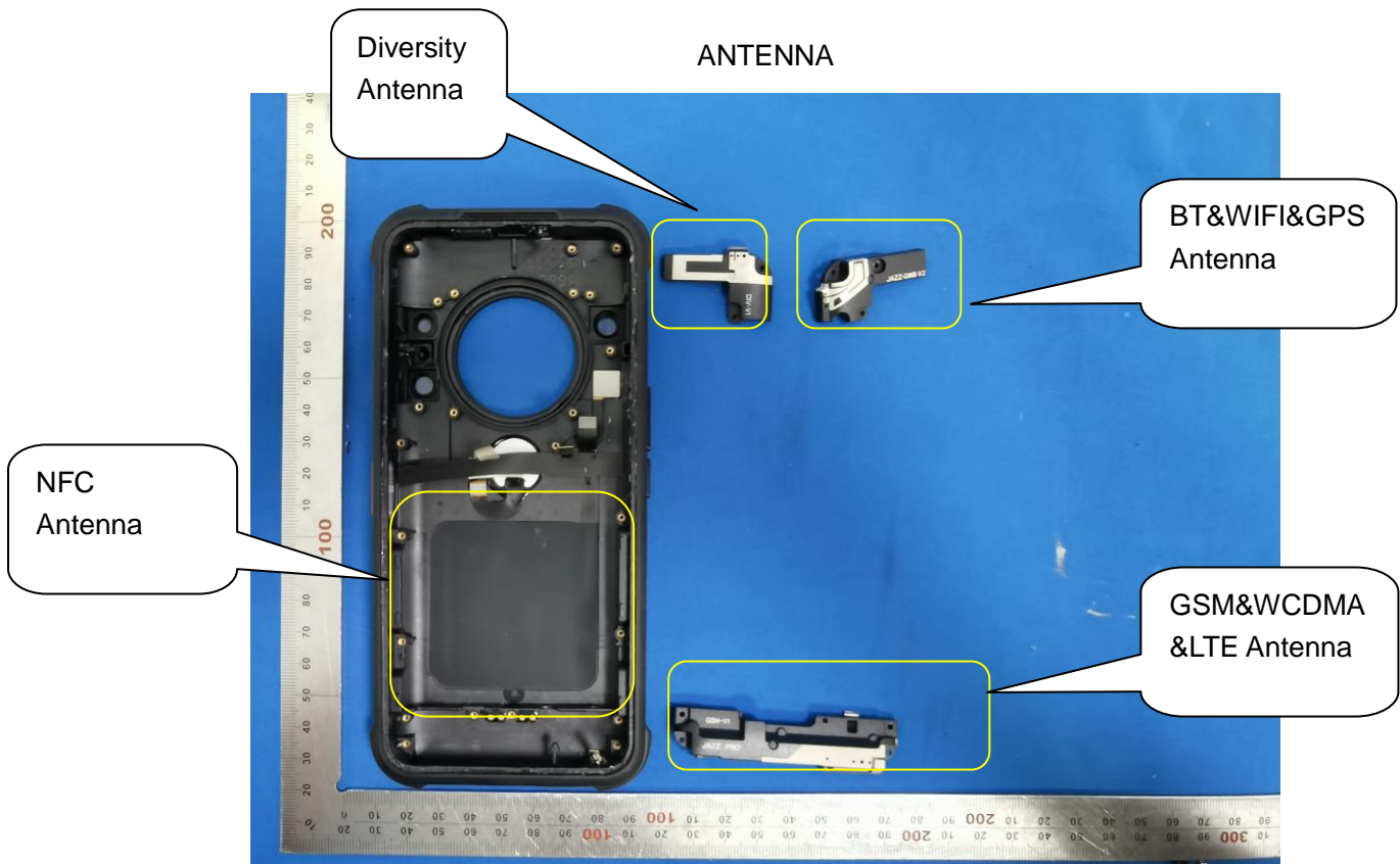
GSM&WCDMA&LTE ANTENNA
