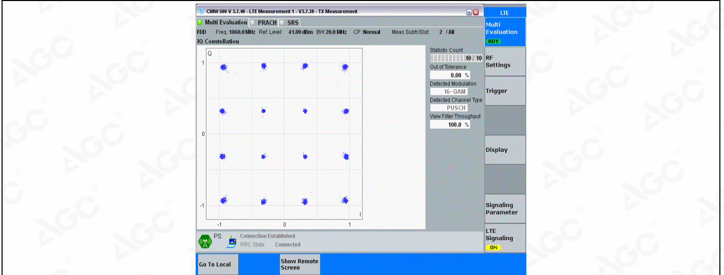
Band25-20MHz-16QAM-26365-100RB#0
