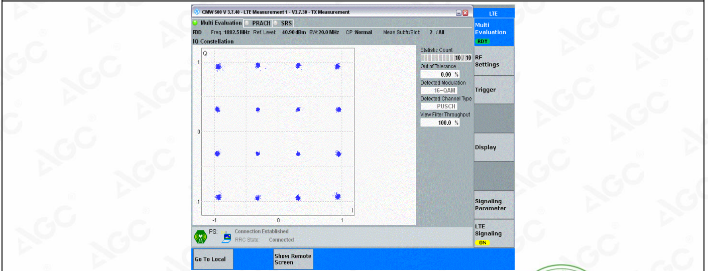
Band25-20MHz-16QAM-26365-100RB#0
