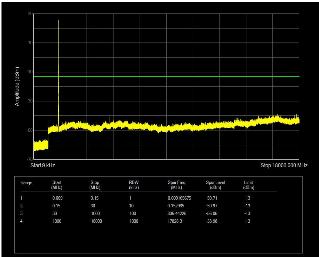
n66 SCS=15kHz CP_QPSK BW=15MHz Channel=354500 RB=1@0
