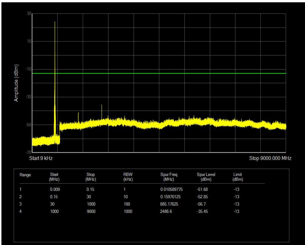
n5 SCS=15kHz CP_QPSK BW=5MHz Channel=165300 RB=25@0
