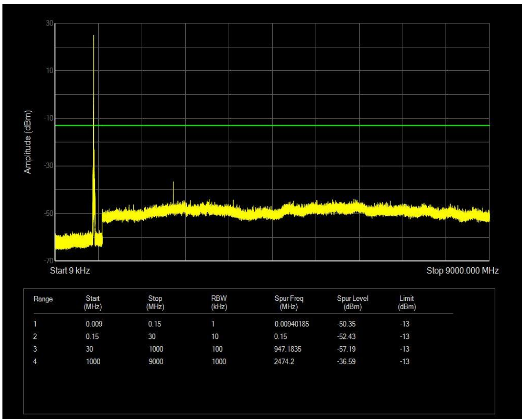
n5 SCS=15kHz CP_QPSK BW=20MHz Channel=166800 RB=1 @105
