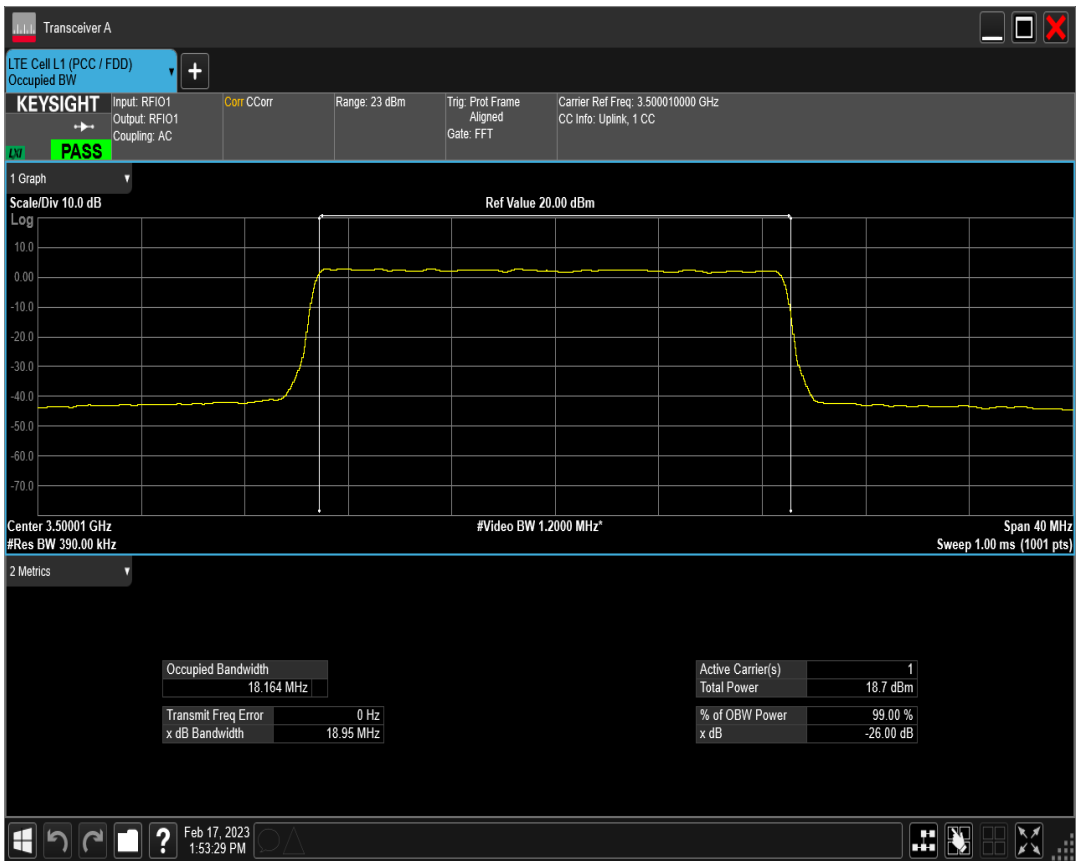
n78(3450-3550) SCS=30kHz DFT 16QAM BW=20MHz Channel=633334 RB=50@0
