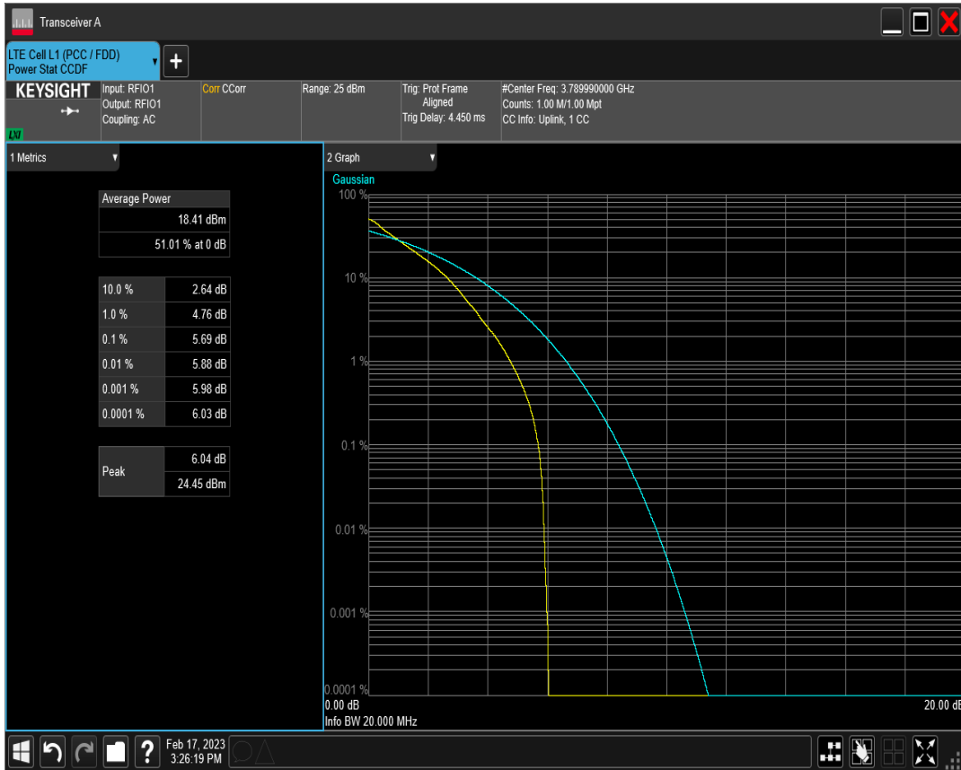
n78(3700-3800) SCS=30kHz DFT 16QAM BW=20MHz Channel=652666 RB=50@0
