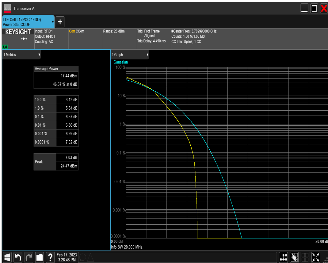
n78(3700-3800) SCS=30kHz DFT 64QAM BW=20MHz Channel=652666 RB=50@0
