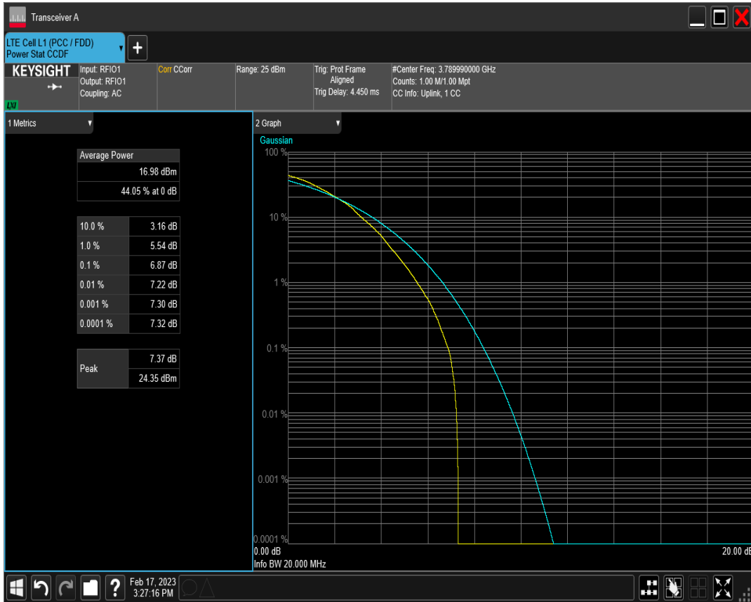
n78(3700-3800) SCS=30kHz DFT 256QAM BW=20MHz Channel=652666 RB=50@0
