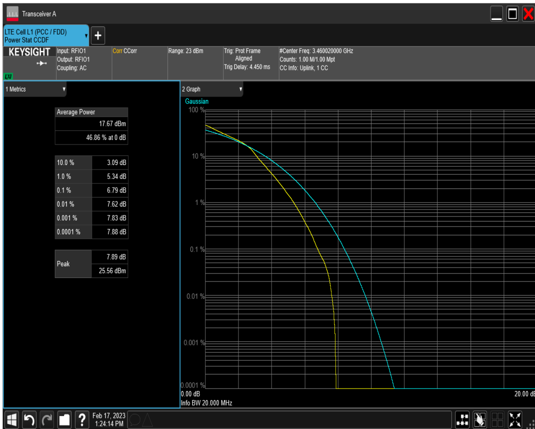
n78(3450-3550) SCS=30kHz DFT 64QAM BW=20MHz Channel=630668 RB=50@0
