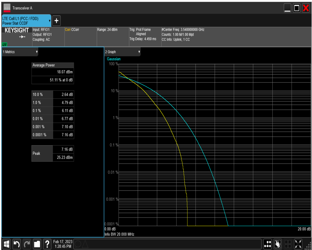
n78(3450-3550) SCS=30kHz DFT 16QAM BW=20MHz Channel=636000 RB=50@0
