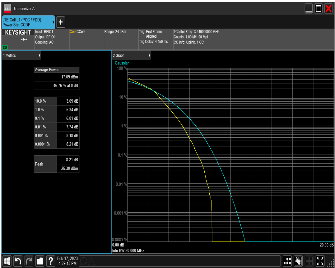
n78(3450-3550) SCS=30kHz DFT 64QAM BW=20MHz Channel=636000 RB=50@0
