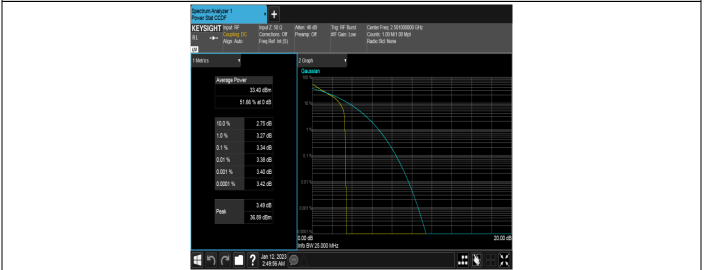
Band41-10MHz-QPSK-39700-50RB#0
