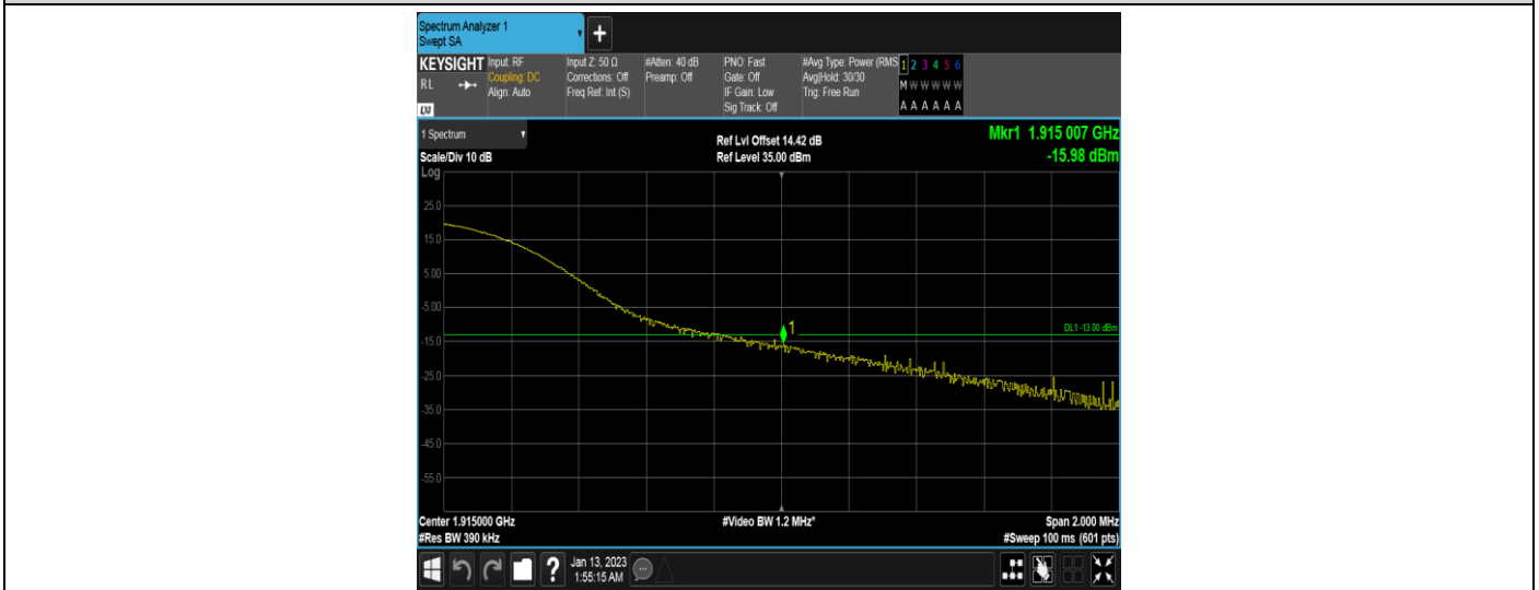
Band25-20MHz-QPSK-26590-1RB#99
