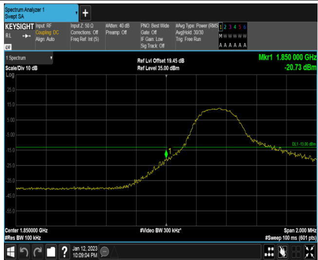
Band2-5MHz-QPSK-18625-1RB#0
