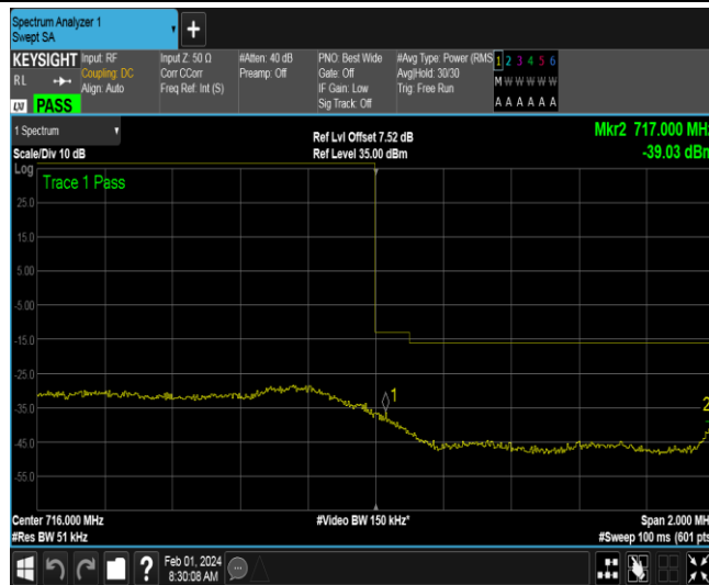
Band12-3MHz-QPSK-23165-1RB#14
