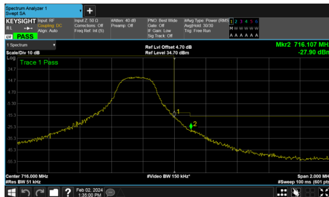
Band12-3MHz-QPSK-23165-15RB#0
