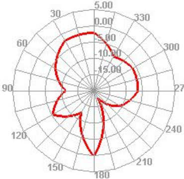
1575.000MHz E1
