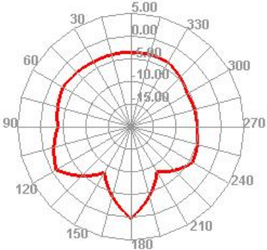
1575.000MHz E2
