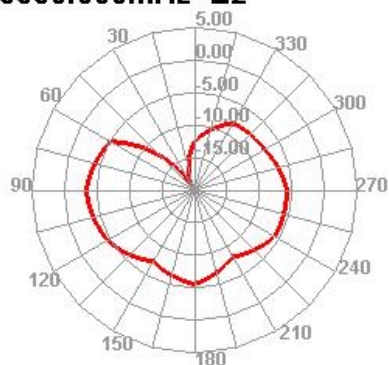
5550.000MHz E2
