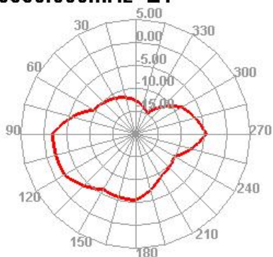
5550.000MHz E1
