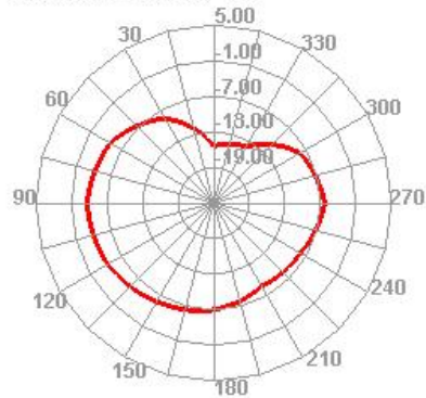
1600.000MHz E2
