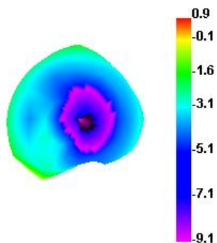
2450.000MHz
