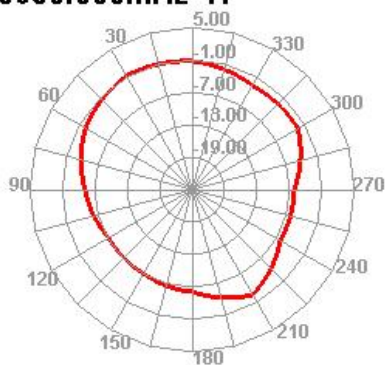
5650.000MHz H
