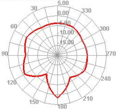
1550.000MHz E2
