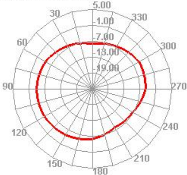
1550.000MHz H
