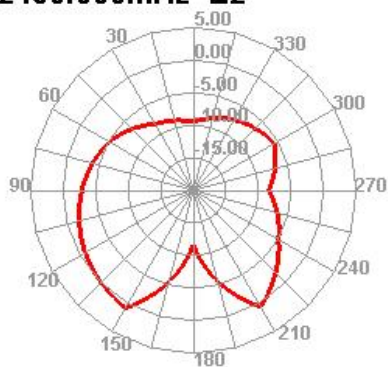
2450.000MHz E2
