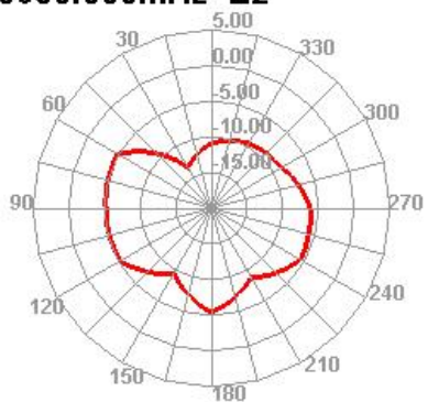
5650.000MHz E2
