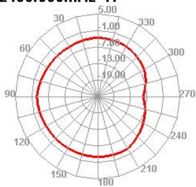
2450.000MHz H
