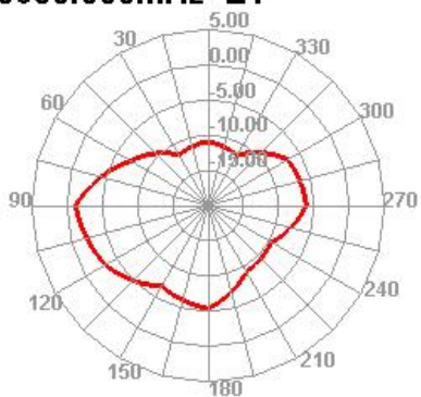
5650.000MHz E1
