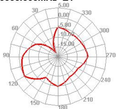
5850.000MHz E1
